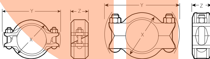
TAMAÑOS CONVENCIONALES DE 1 ½ – 4"/40 – 100 mm
