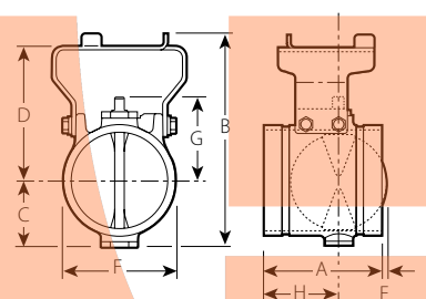
TAMAÑOS CONVENCIONALES DE 2 1/2 – 3”/66,7 – 79,4 mm
