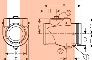
TAMAÑOS CONVENCIONALES DE 4 – 8"/100 – 200 mm
