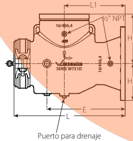
TAMAÑOS DE 14" – 24" / 350-600 MM
