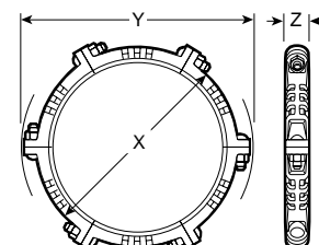
TAMAÑOS DE 24 – 36"/600 – 900 mm
