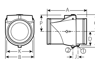
TAMAÑOS CONVENCIONALES DE 10 – 12"/250 – 300 mm
