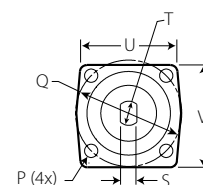
BRIDA DE MONTAJE EXPANDIDA TÍPICO DE TAMAÑOS 2 - 8" / 50 - 200 mm (LA VÁLVULA APARECE CERRADA)
