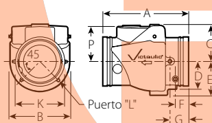
TAMAÑOS CONVENCIONALES DE 4"/100 mm
