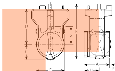
TAMAÑOS CONVENCIONALES DE 4 – 5”/104,8 – 130,2 mm
