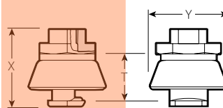
TAMAÑOS CONVENCIONALES DE 10"/250 mm Y MAYORES
