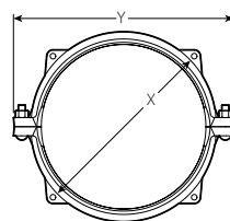
TAMAÑOS CONVENCIONALES DE 26-60"/660-1525 MM
