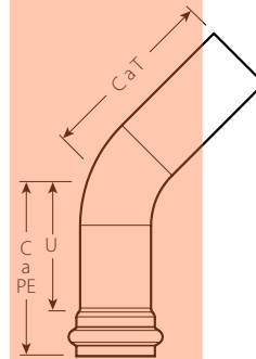
ESTILO P543 Y P563
