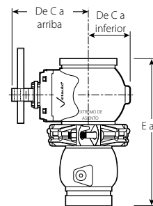
TAMAÑO CONVENCIONAL DE 3"/80 mm
