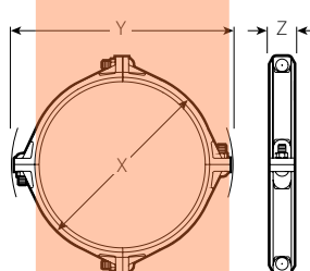
TAMAÑOS CONVENCIONALES DE 14 – 20"/350 – 500 mm
