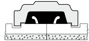
TUBERÍA CON REVESTIMIENTO DE CEMENTO
