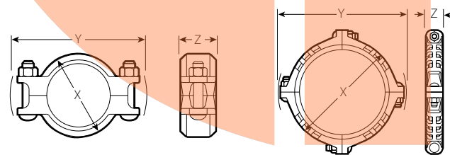
TAMAÑOS CONVENCIONALES DE 3/4 – 14"/20 – 350 mm
