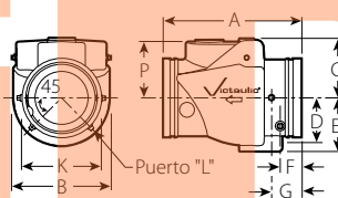
TAMAÑOS CONVENCIONALES DE 5 – 6"/125 – 165,1 mm
