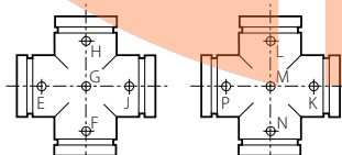
CONEXIÓN EN CRUZ – TAMAÑO RECTO
