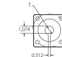
BRIDA DE MONTAJE EXPANDIDA TÍPICO DE TAMAÑOS DE 10" / 250 mm (LA VÁLVULA APARECE CERRADA)
