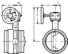
VÁLVULA CON PALANCA DE ACCIONAMIENTO DE ENGRANAJES. TAMAÑOS CONVENCIONALES DE 2 – 8"/50 – 165,1 mm
