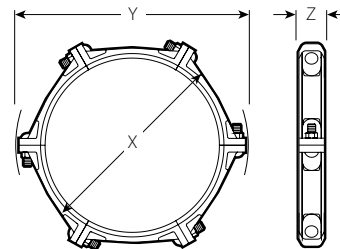
TAMAÑOS CONVENCIONALES DE 24 – 36"/600 – 900 mm
