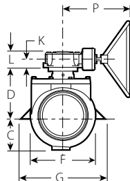
TAMAÑOS CONVENCIONALES DE 8 – 12"/200 – 300 MM
