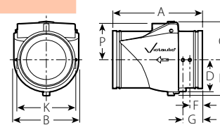
TAMAÑOS CONVENCIONALES DE 8 – 12"/200 – 300 mm
