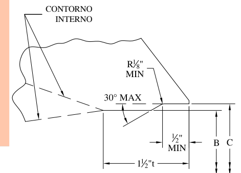
Fig. 2.- Preparación de extremos soldables para ensamblar con arillo de respaldo rectangular continuo (contorno interno)
